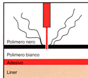
Materiale per incisione laser codice prodotto 7847
